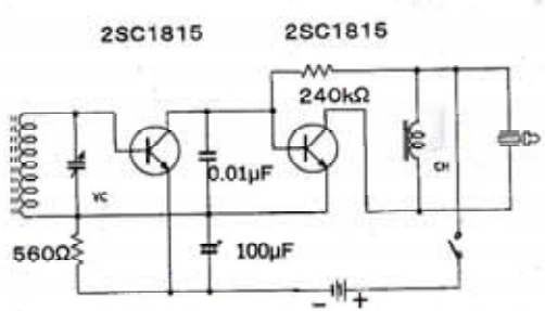
2石トランジスタラジオ回路図
